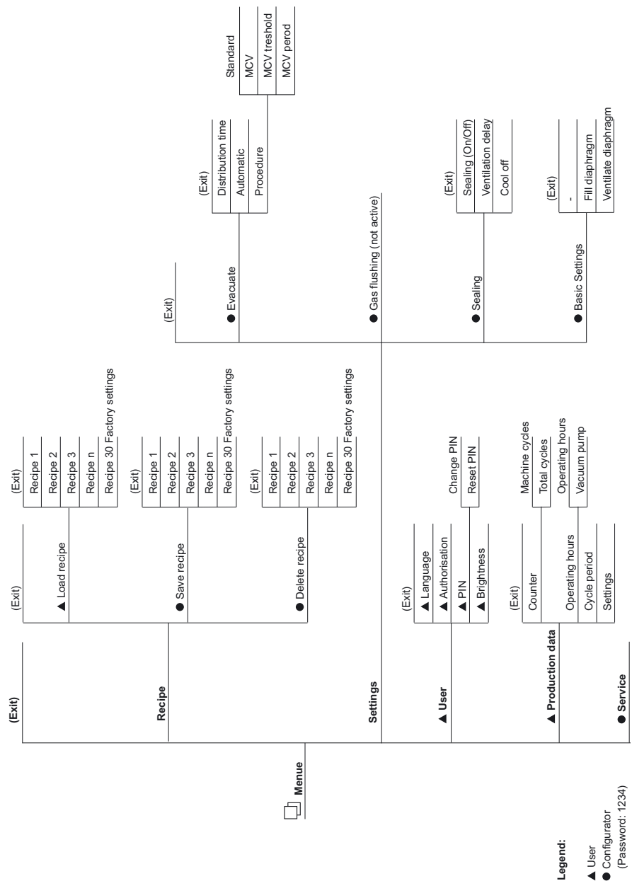
Рис. 22: Структура меню
